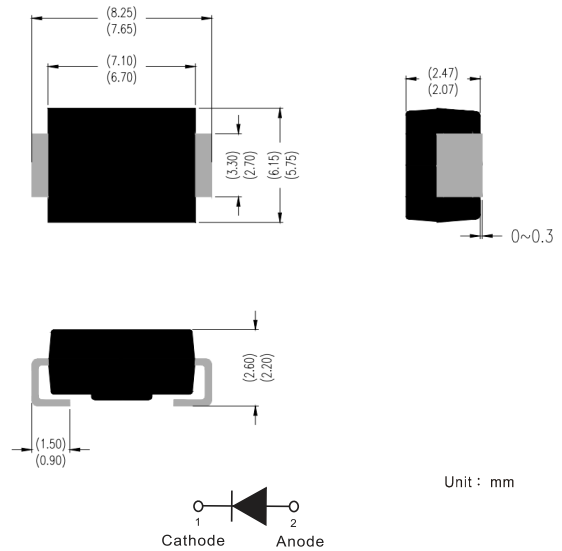
DO-214AB (SMC)
